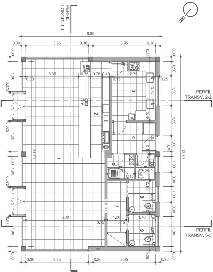
PLANTA DO PISO
