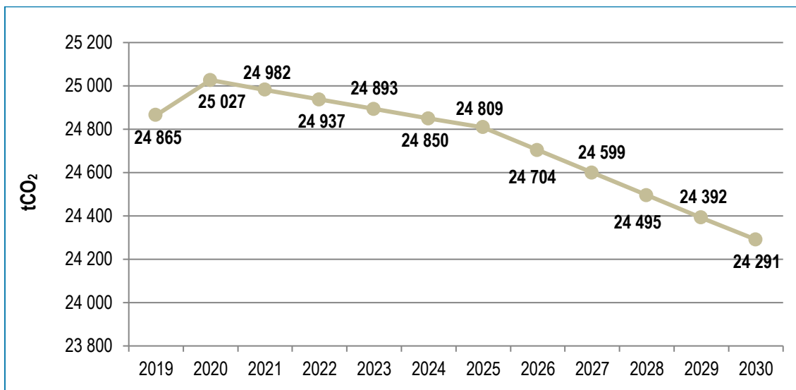
Figura 22. Emissões de GEE no Município de Tomar: Setor dos Serviços (2019-2030)
