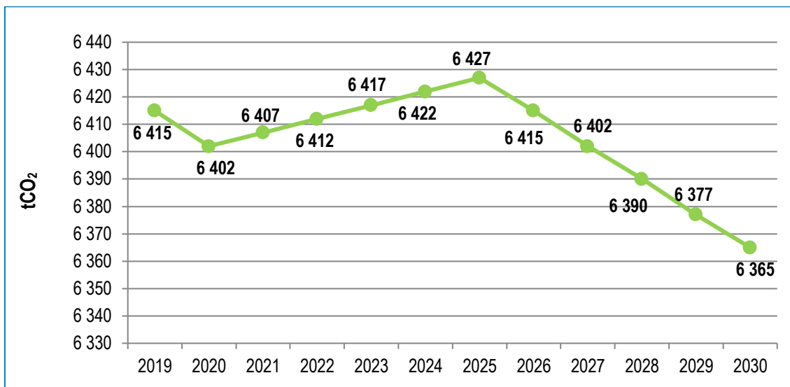
Figura 24. Emissões de GEE no Município de Tomar: Setor da Agricultura (2019-2030)
