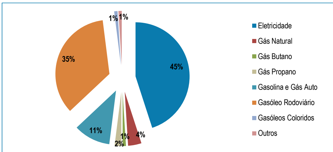
Figura 19. Emissões de GEE por Vetor Energético no Município de Tomar (2030)
