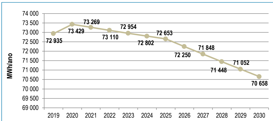
Figura 14. Consumos de energia no Município de Tomar: Setor dos Serviços (2019-2030)
