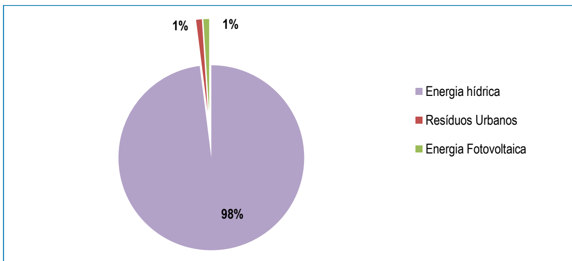
Figura 26. Repartição da produção renovável de energia no concelho de Tomar, por fonte energética (2016)
