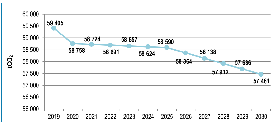
Figura 25. Emissões de GEE no Município de Tomar: Setor dos Transportes (2019-2030)
