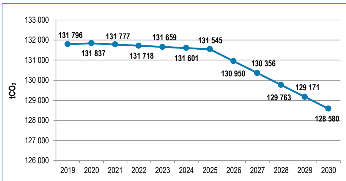
Figura 18. Emissões de GEE no Município de Tomar (2019-2030)
