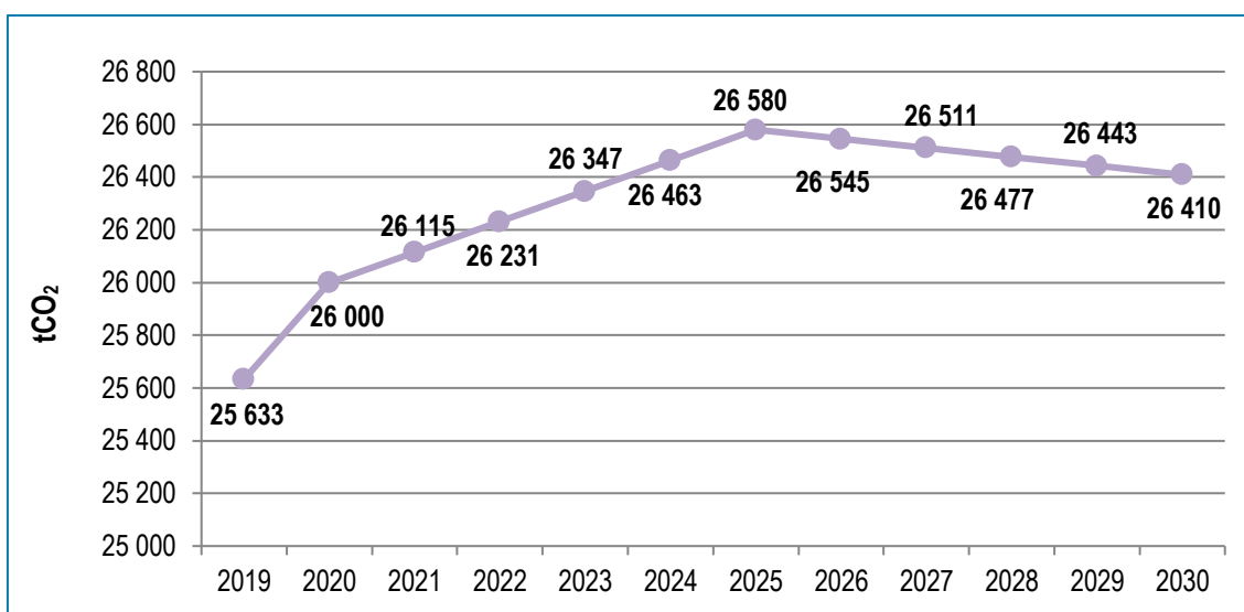
Figura 21. Emissões de GEE no Município de Tomar: Setor Doméstico (2019-2030)
