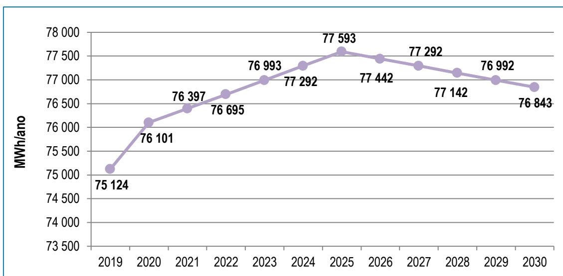
Figura 13. Consumos de energia no Município de Tomar: Setor Doméstico (2019-2030)
