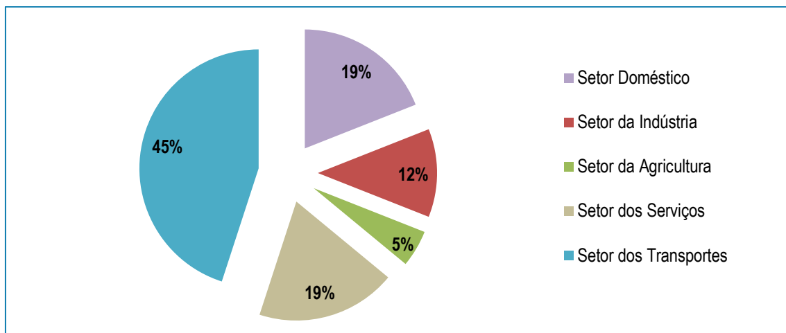
Figura 20. Emissões de GEE no Município de Tomar, por setor (2019)
