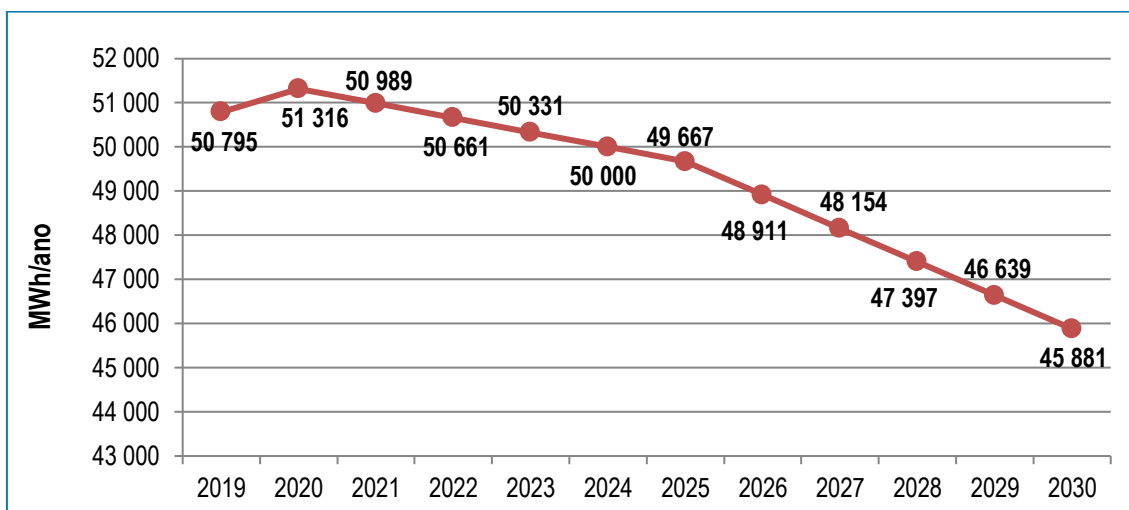
Figura 15. Consumos de energia no Município de Tomar: Setor da Indústria (2019-2030)
