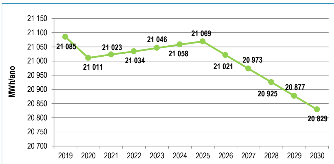
Figura 16. Consumos de energia no Município de Tomar: Setor da Agricultura (2019-2030)
