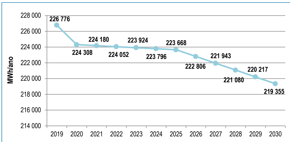
Figura 17. Consumos de energia no Município de Tomar: Setor dos Transportes (2019-2030)
