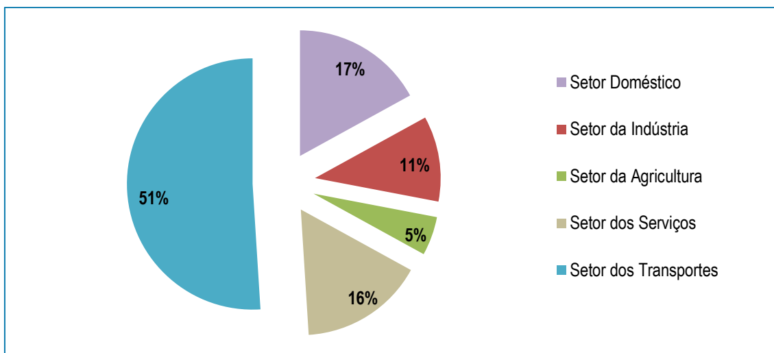
Figura 12. Consumos de energia no Município de Tomar, por setor (2019)
